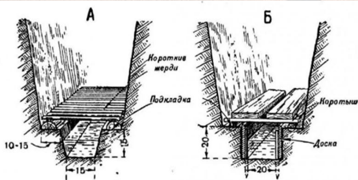
Рис. 32. Осушение дна окопа:
